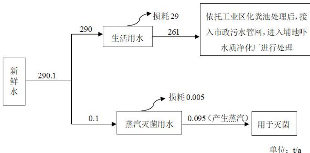
图 2-7 项目水平衡图
